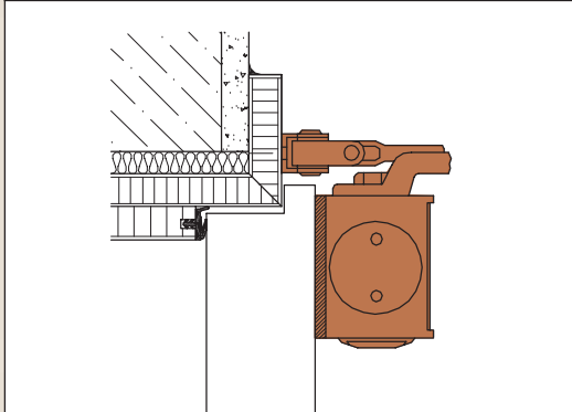
SCHERENARMTÜRSCHLIEßER
