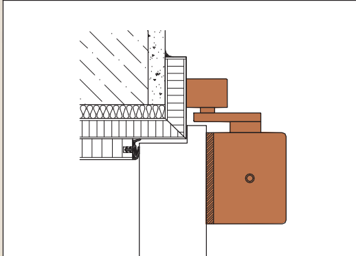
GLEITSCHIENENTÜRSCHLIEßER
