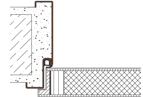
FEUERSCHUTZTÜR AHS TYP 1 MIT STAHLZARGE
